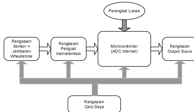
Gambar 2. Diagram blok termometer suara
