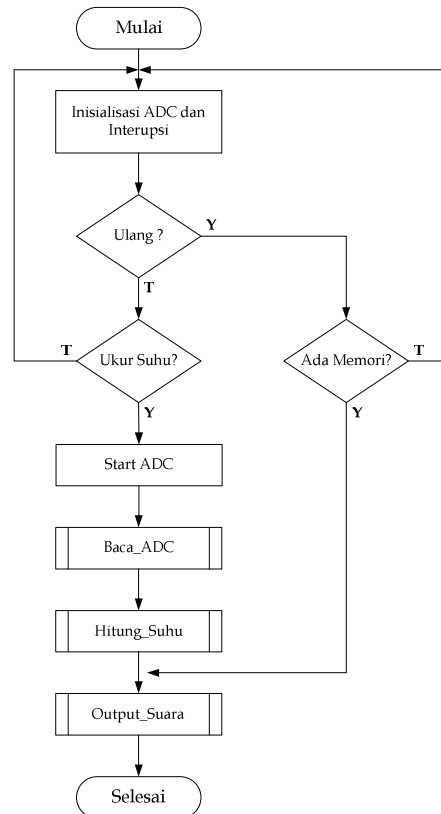
Gambar 8. Diagram alir program utama mikrokontroler
