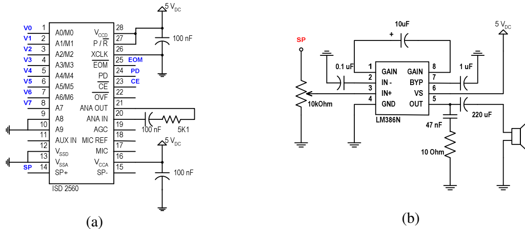
Gambar 5. (a) Rangkaian pemutar suara ; (b) Rangkaian penguat audio
