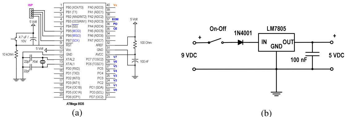
Gambar 6. (a) Rangkaian mikrokontroler ATmega 8535; (b) Rangkaian catu daya
