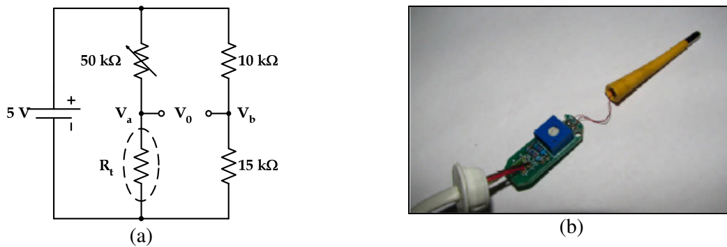
Gambar 3. Skematik (a) dan realisasi (b) rangkaian sensor dan Jembatan Wheatstone
