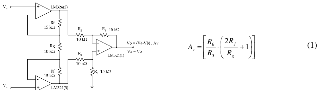
Gambar 4. Rangkaian dan persamaan penguatan penguat instrumentasi [1]
