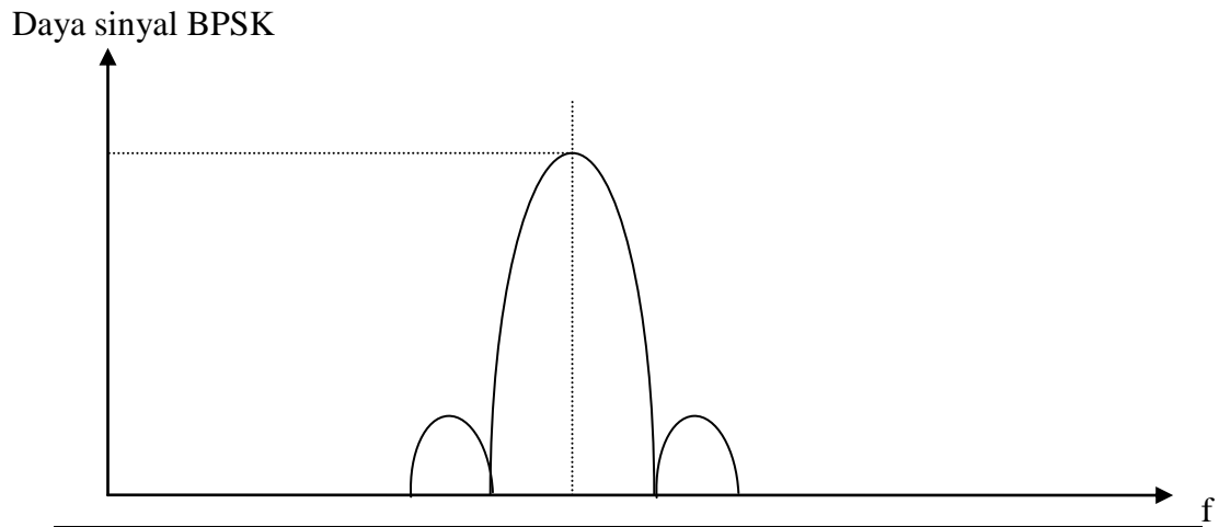
Gambar 5a. Sinyal informasi (BPSK) Sebelum ditebarkan
