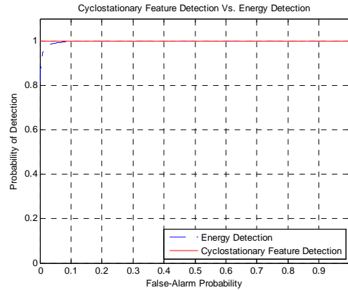
Gambar 9. Kinerja dengan SNR = 12 dB
