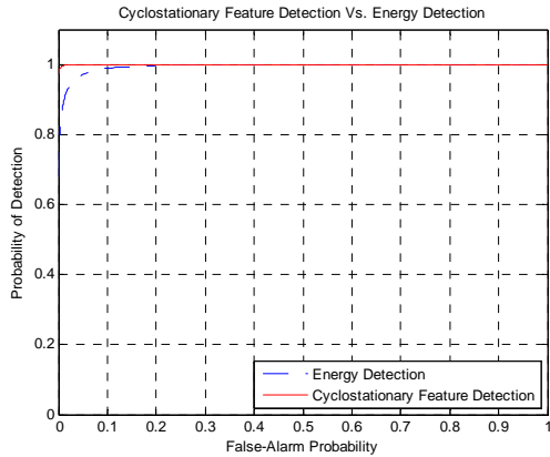
Gambar 8. Kinerja dengan SNR = 11 dB
