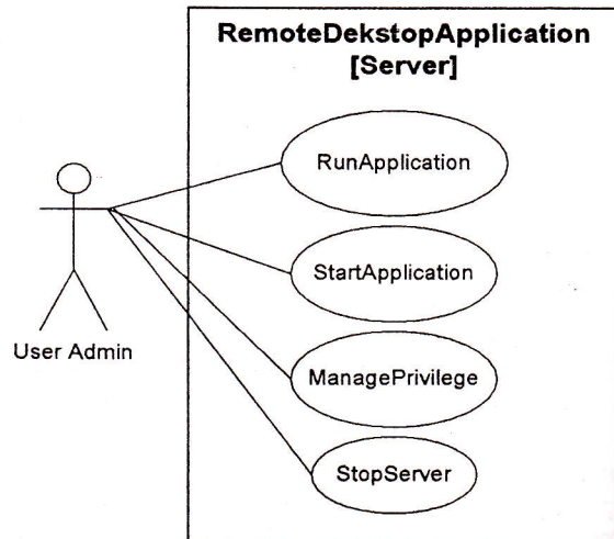
Gambar 2. Use case diagram Remote Dekstop pada bagian Server
