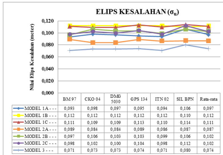
Gambar 8. Grafik perbandingan elips kesalahan
