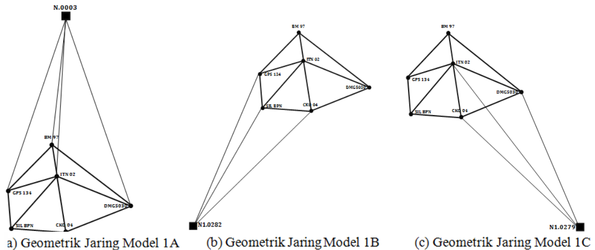
Gambar 2. Geometrik jaring hitungan model 1
