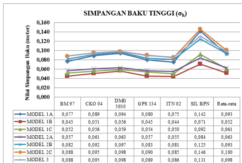
Gambar 9. Grafik Perbandingan simpangan baku tinggi
