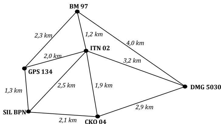
Gambar 1. Geometrik jaring segitiga
