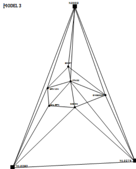
Gambar 4. Geometrik jaringan hitungan model 3
