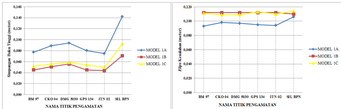
Gambar 6. Grafik simpangan baku tinggi dan elips kesalahan hitungan model 1
