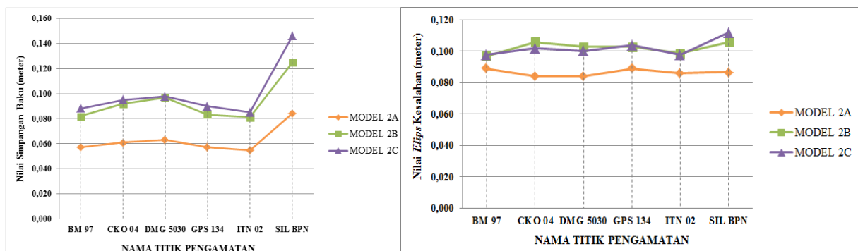
Gambar 7. Grafik simpangan baku dan elips kesalahan hitungan model 2
