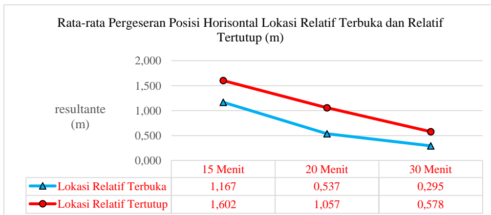
Gambar 9. Grafik Pergeseran Titik Berdasarkan Ruang Pandang ke Langit
