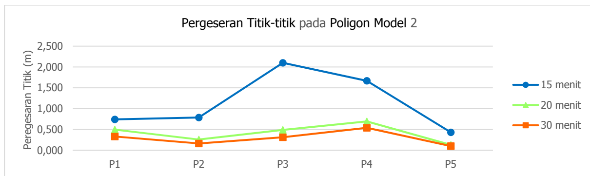
Gambar 6. Grafik Pergeseran Posisi Horisontal Titik-titik pada Poligon Model 2
