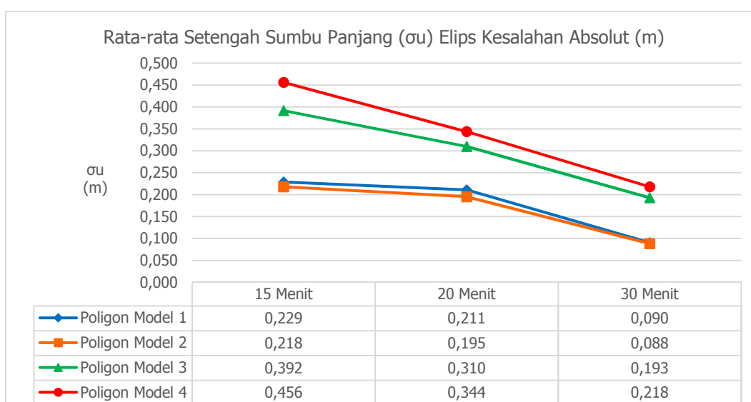
Gambar 3. Grafik Rata-rata Elips Kesalahan Absolut
