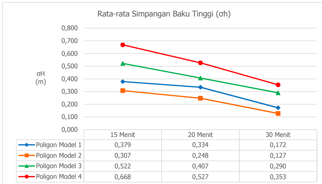
Gambar 4. Grafik Ketelitian Tinggi Rata-rata
