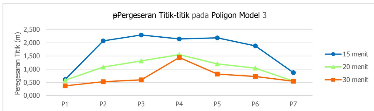
Gambar 7. Grafik Pergeseran Posisi Horisontal Titik-titik pada Poligon Model 3
