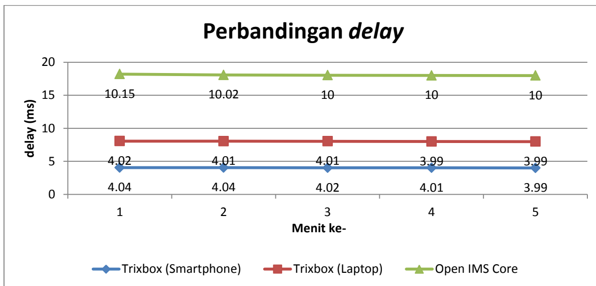
Gambar 4. Perbandingan delay
